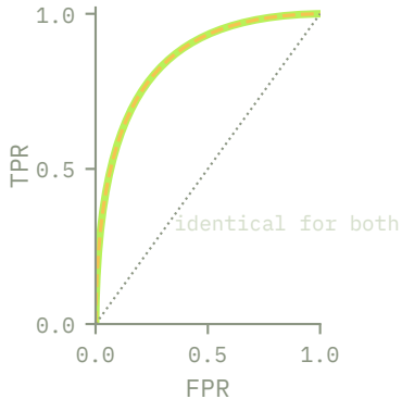
ROC
