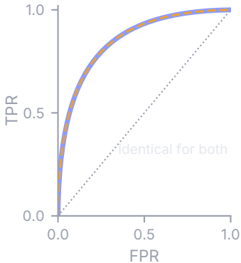
ROC
