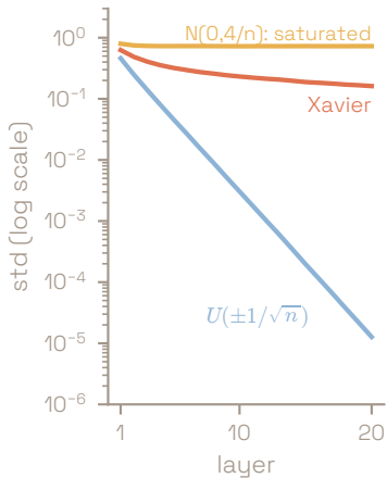
tanh layers
