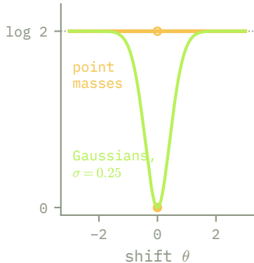
JSD (nats)
