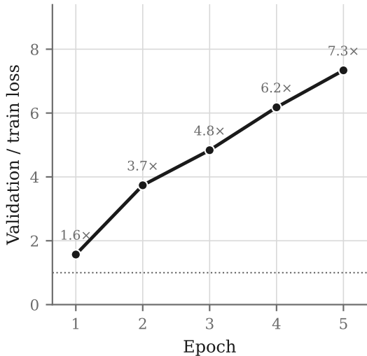
(b) Generalisation gap
