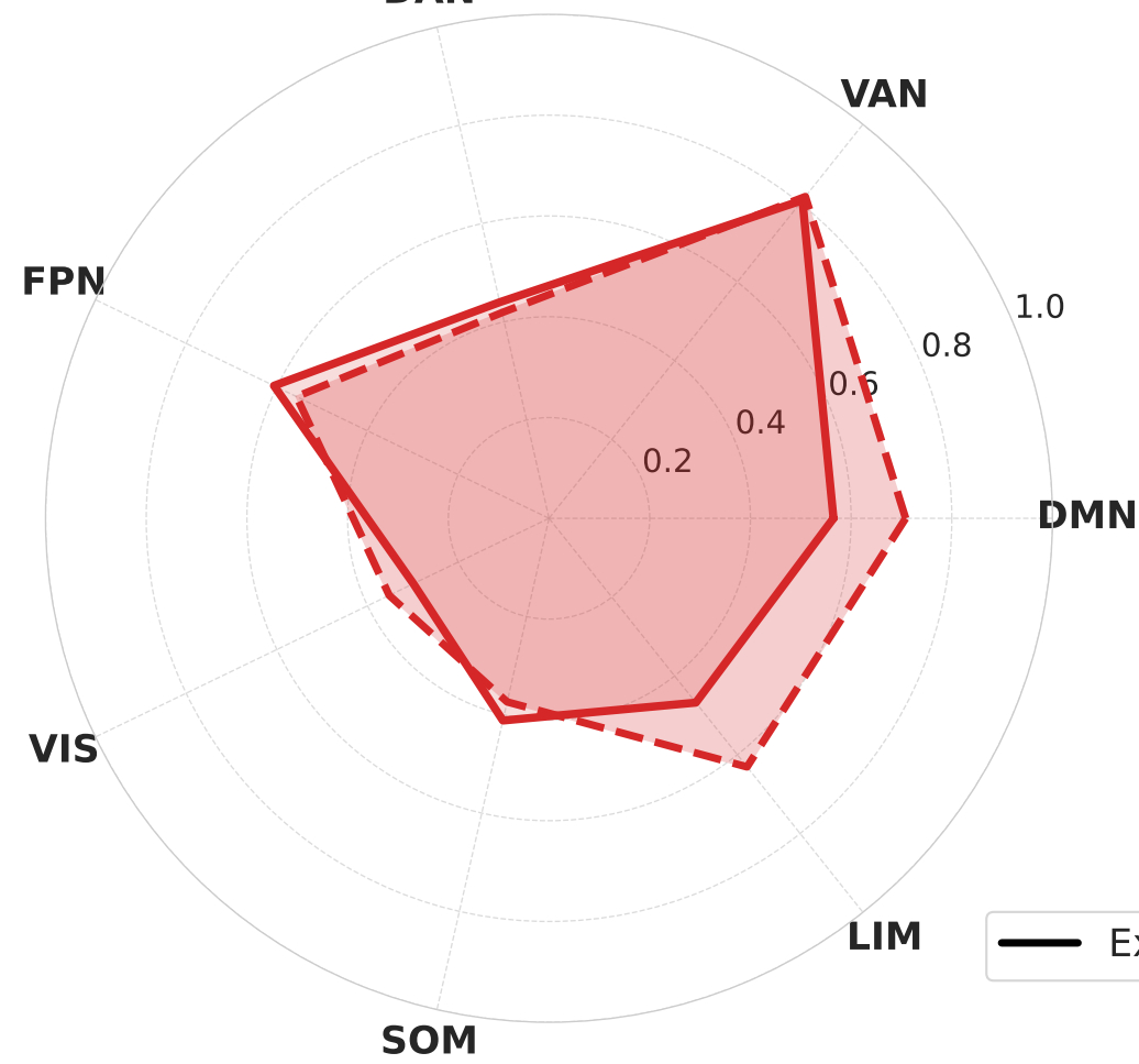
Meta Awareness DAN
