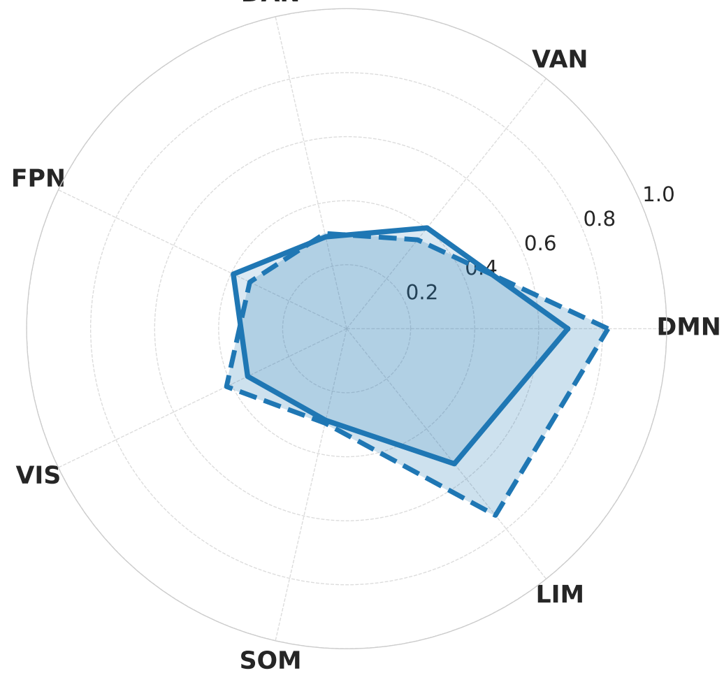
Mind Wandering DAN
