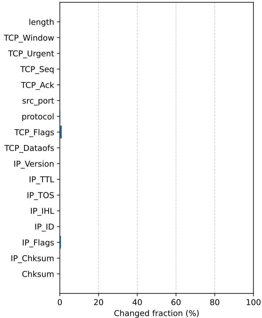
Knn
