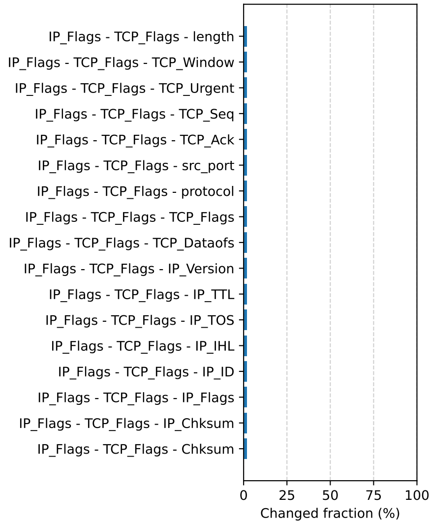
Knn
