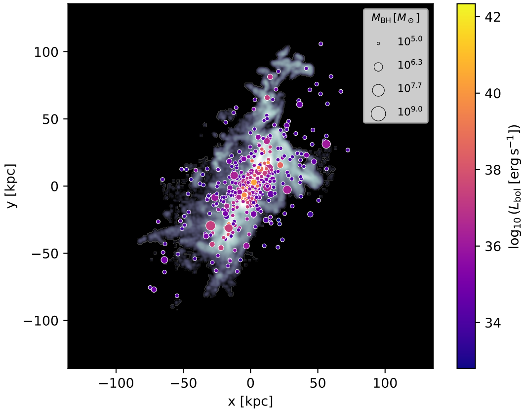
z=0.30 : subhalo 1, 395 BH(s)
