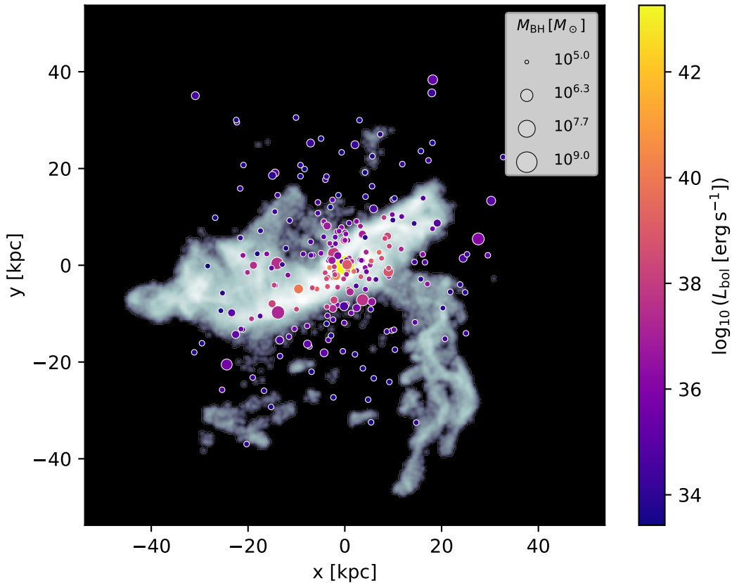
z=0.20 : subhalo 1, 223 BH(s)
