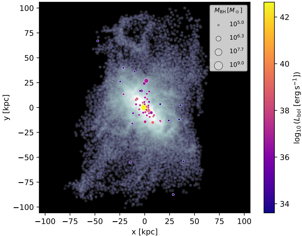
z=0.00 : subhalo 3344, 56 BH(s)
