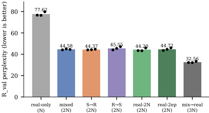
N = 1M real tokens
