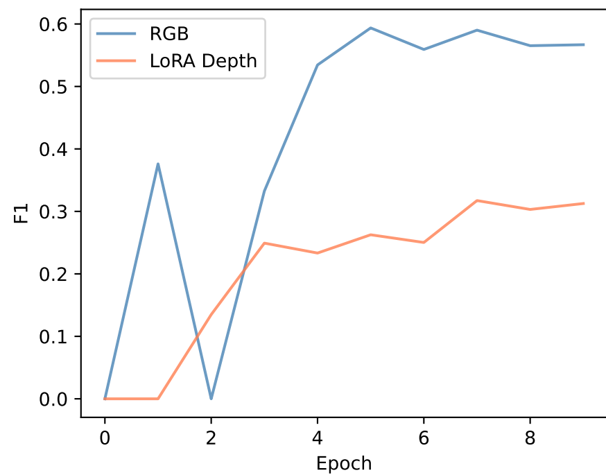
Validation F1
