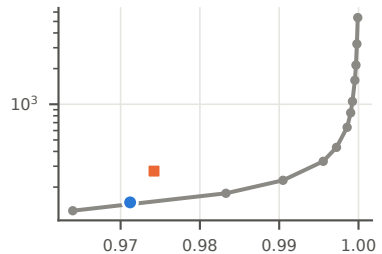
Last.fm (x-modal) · KS 0.216
