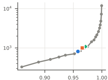
DeepImage-96 · KS 0.066
