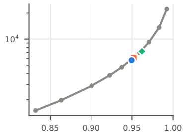
MS MARCO-384 · KS 0.044
