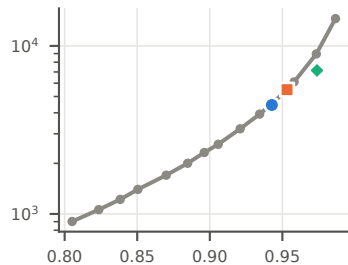
COCO-I2I · KS 0.046
