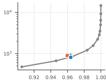
Cohere-1024 · KS 0.049
