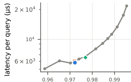
DeepImage-96 · KS 0.066
