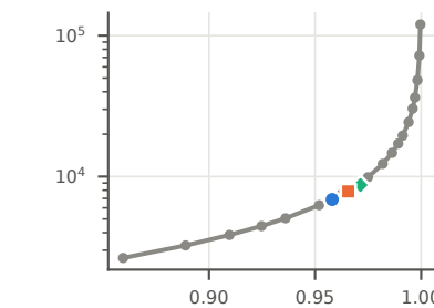
Yambda · KS 0.090
