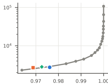
iNat-ResNet · KS 0.115
