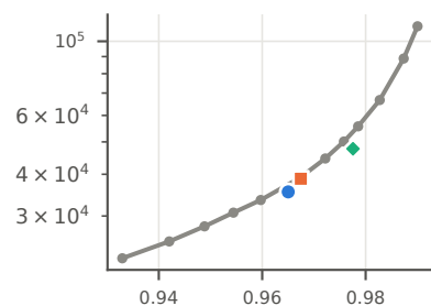
DeepImage-96 · KS 0.066
