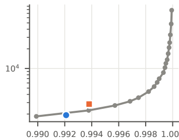
iNat-ResNet · KS 0.115
