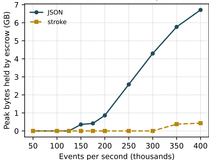
(b) Escrow held, no cap
