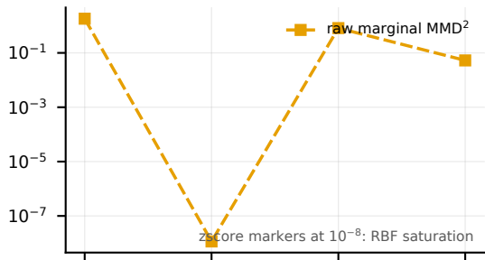
CREMA-D → RAVDESS
