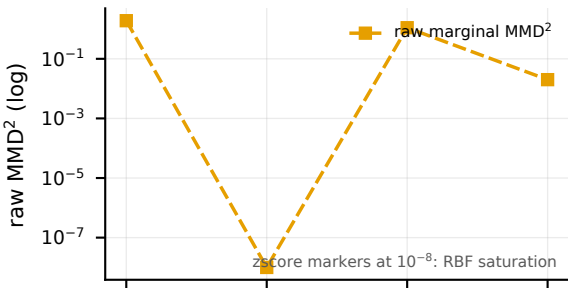
RAVDESS → CREMA-D
