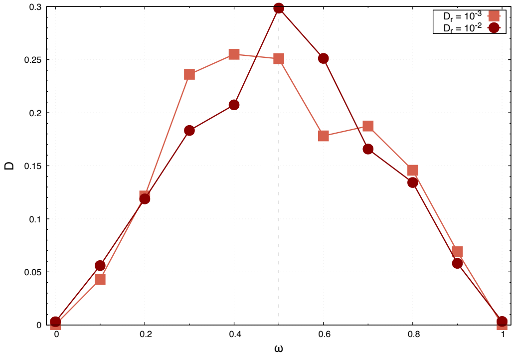
TCRW Fig 1(d) — D(\omega) , T = 10^6 , N_{\text{traj}} = 500
