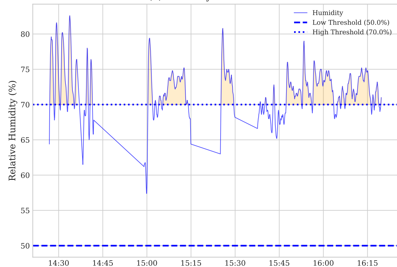
(d) Humidity - MANUAL Mode
