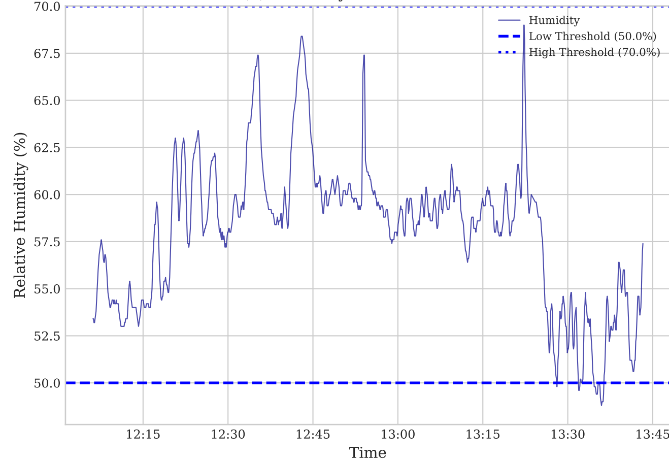
(d) Humidity - MANUAL Mode
