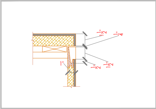
E)DETAIL - A
