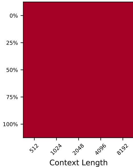
ALiBi
