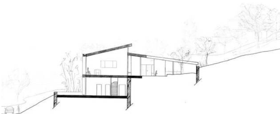
COUPE AA
