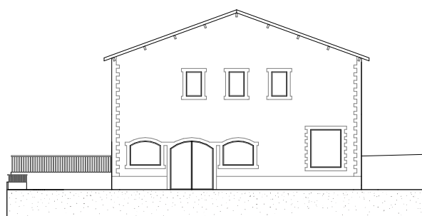
FAÇADE OUEST
