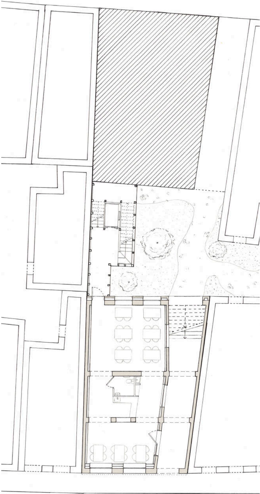
PLAN RDC
