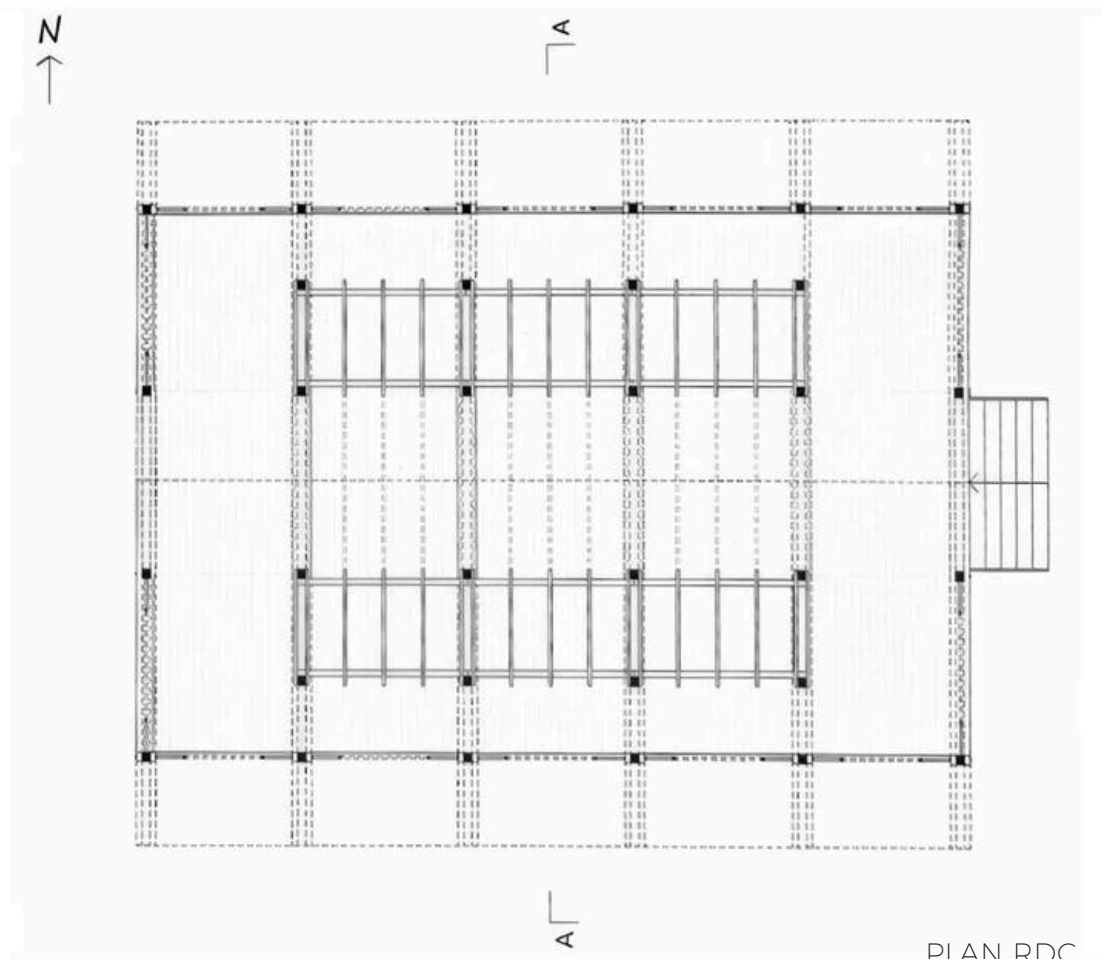
PLAN RDC
