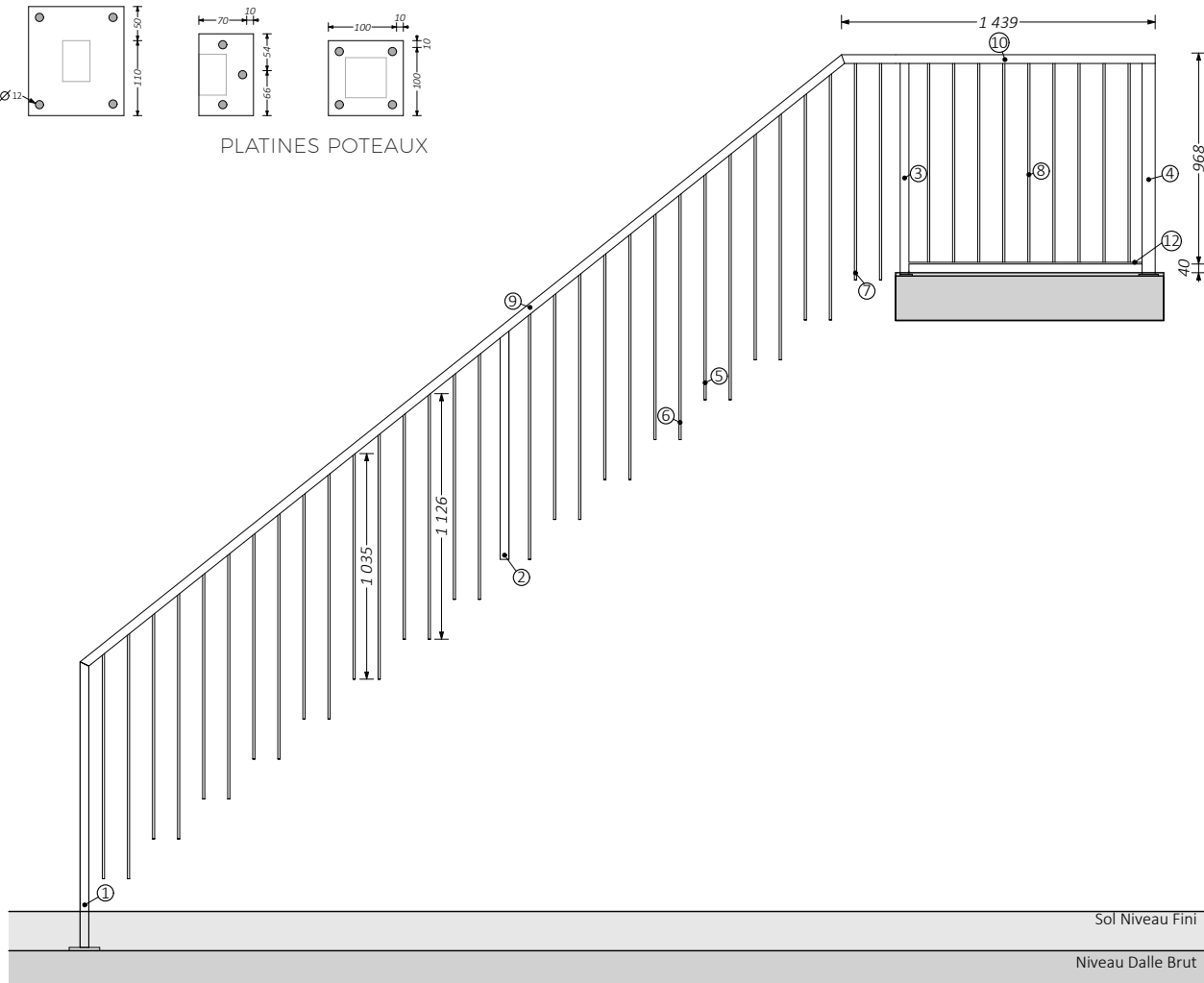
VUE DE FACE GARDE-CORPS
