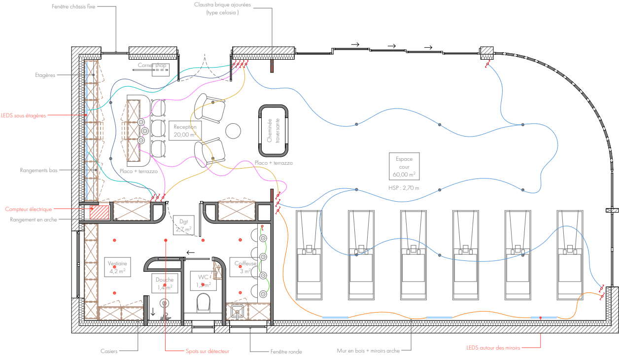
PLAN D'ÉCLAIRAGE
