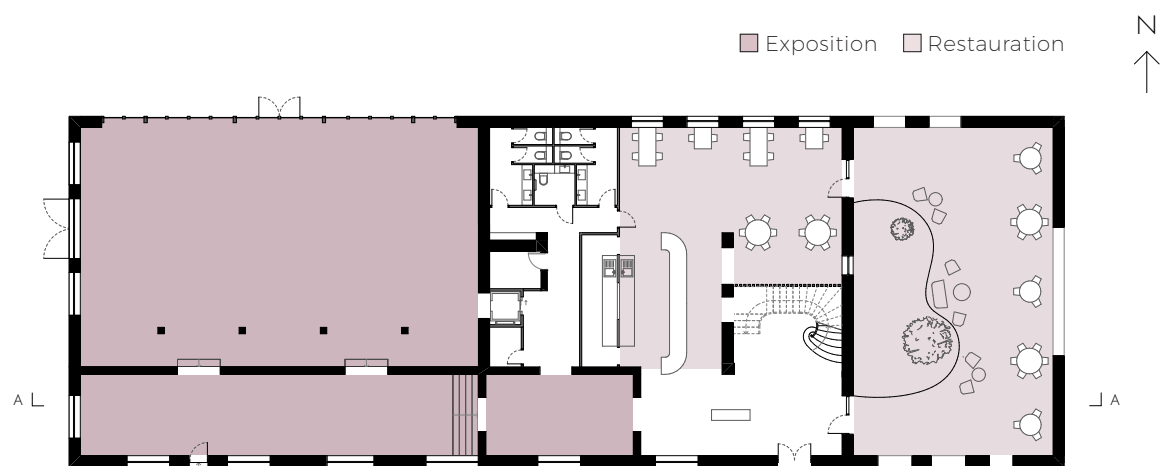
PLAN RDC PROJET
