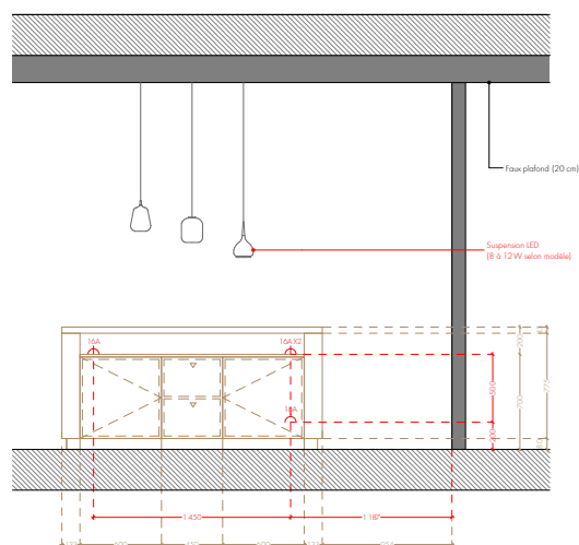
COUPE AA
