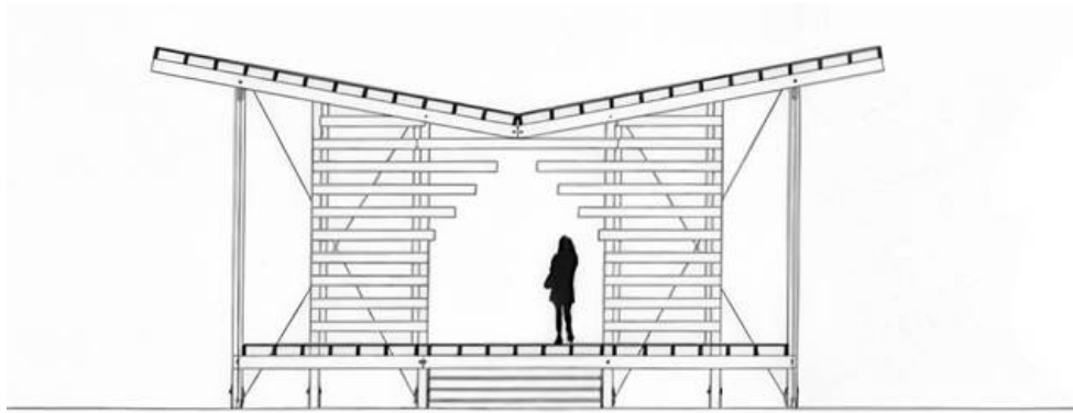
COUPE AA
