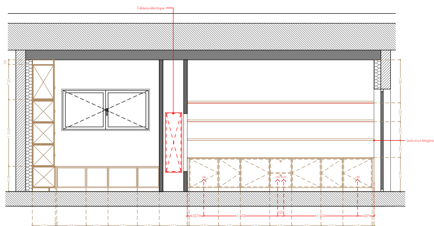
COUPE CC
