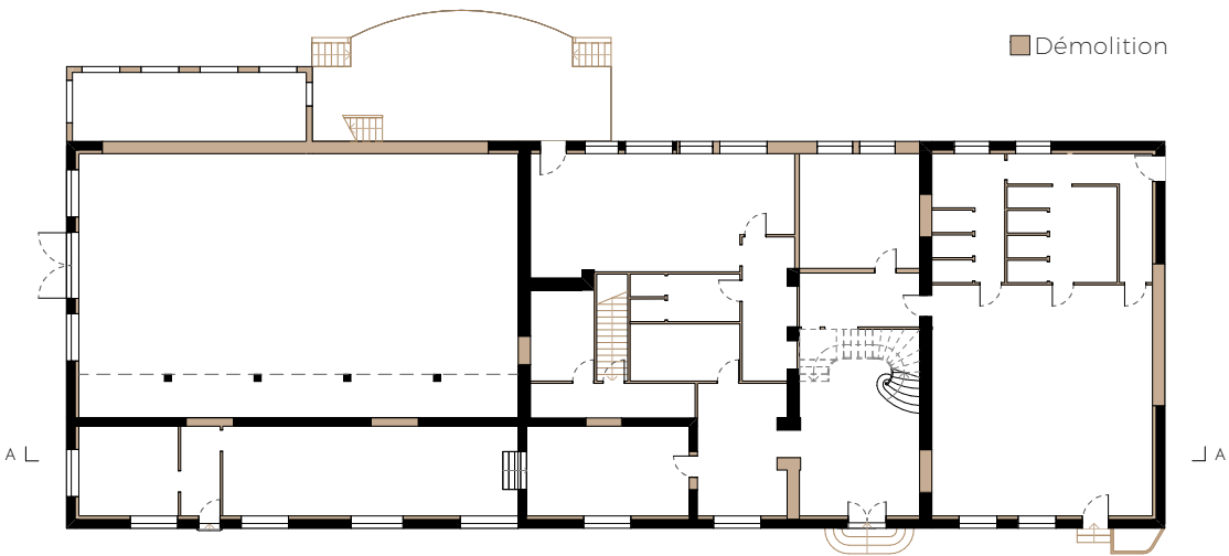
PLAN RDC EXISTANT
