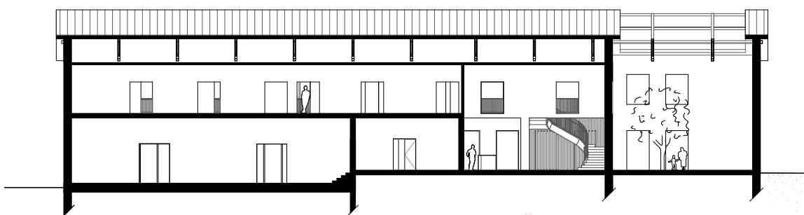
COUPE AA
