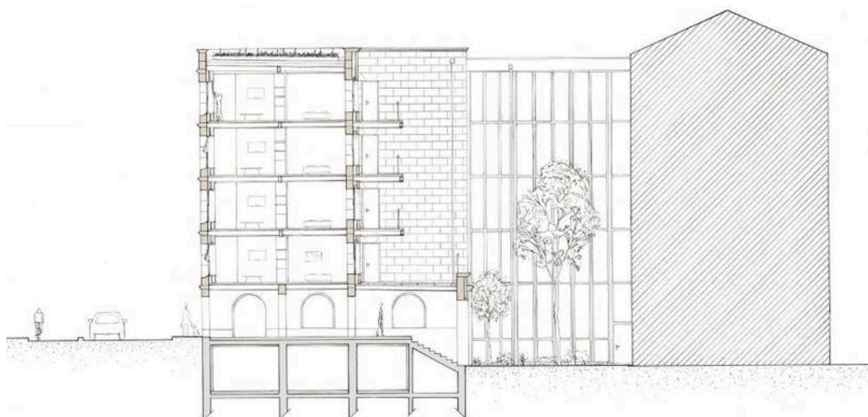
COUPE
