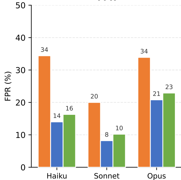
FPR
