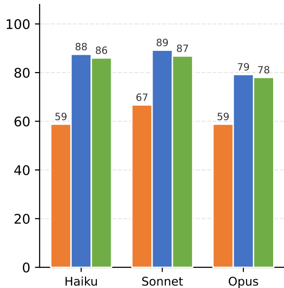
Precision
