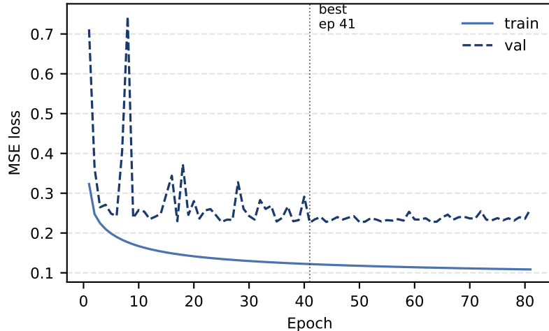
(d) + dropout ( p = 0.1 )
