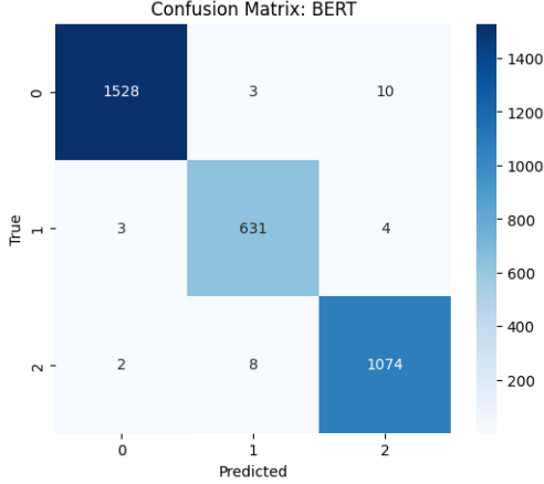
Fig. 3. BERT confusion matrix.
