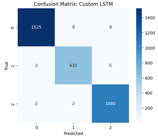
Fig. 1. LSTM confusion matrix.
