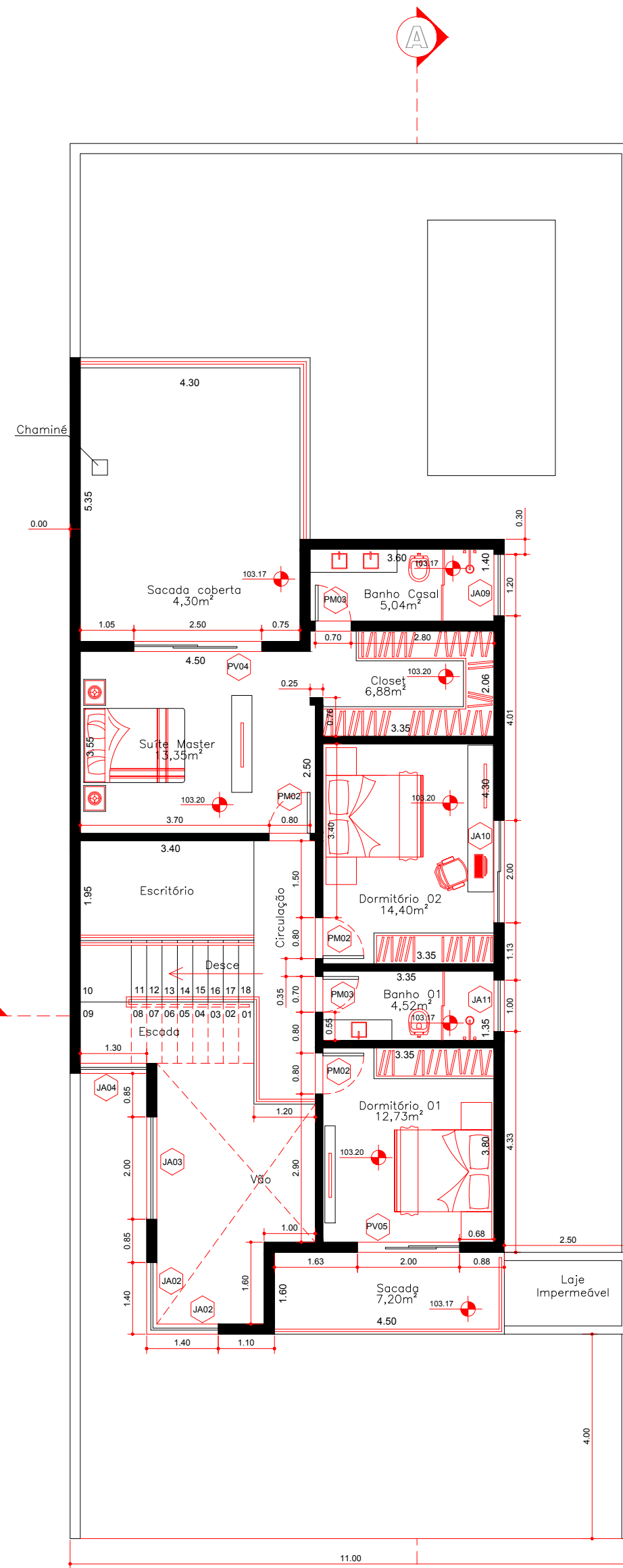
Planta Baixa Superior Escala - 1:100
