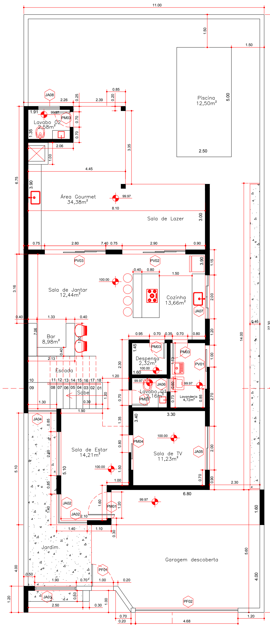
Planta Baixa Térreo Escala - 1:100
