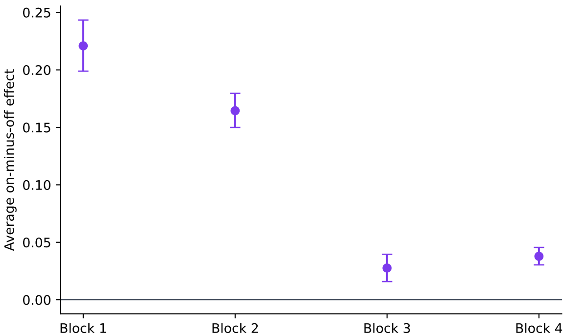
Feature 6779 · harmful
