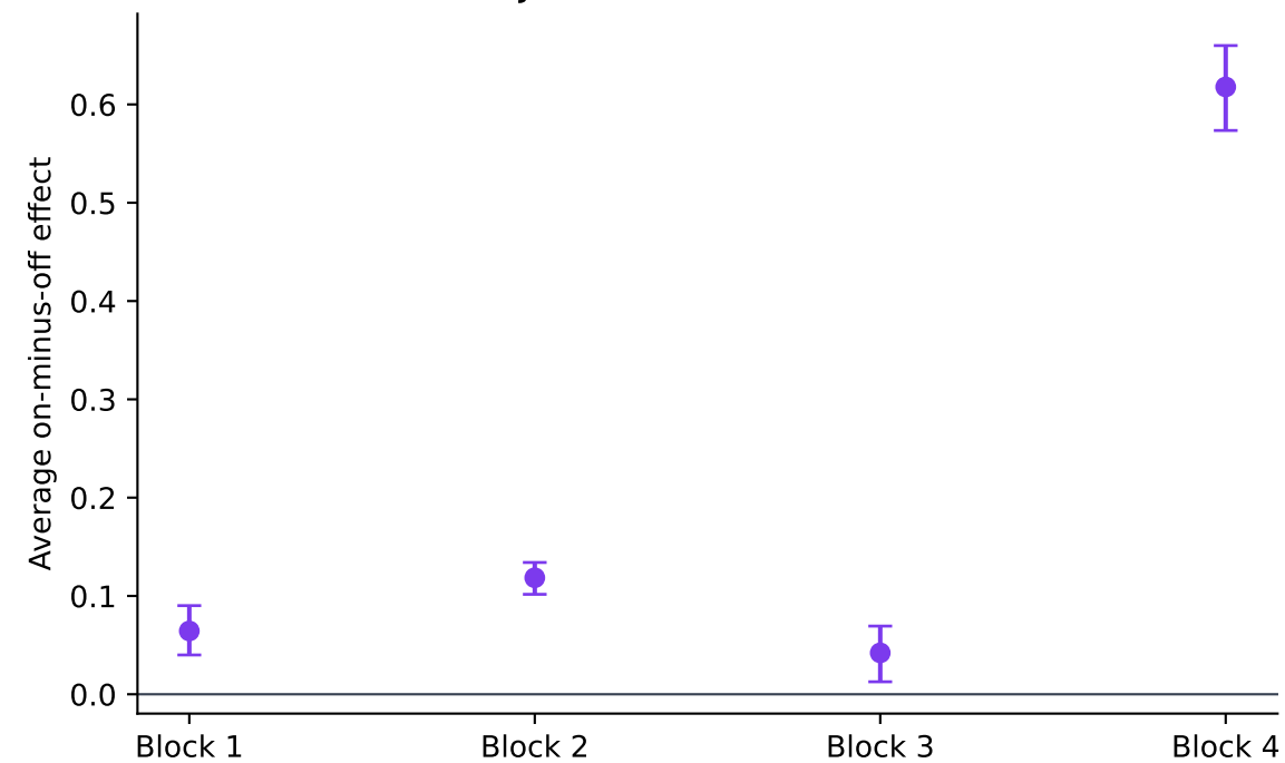
Feature 6779 · harmful
