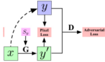
Rysunek 7: Model PoseGAN [1]. Notacje: x i y to rzeczywiste obrazy; y' to wygenerowany obraz; S_y to szkielet y ; G to generator; D to dyskryminator
