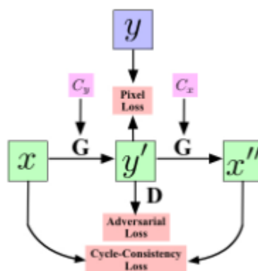
Rysunek 5: Model GestureGAN [6]. Oznaczenia: x i y to rzeczywiste obrazy; x' i y' to wygenerowane obrazy; x'' to zrekonstruowane obrazy; C_x i C_y to kontrolowane struktury, odpowiednio x i y ; G to generator; D to dyskryminator
