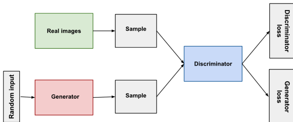
Rysunek 4: Ogólny model sieci GAN [4]
