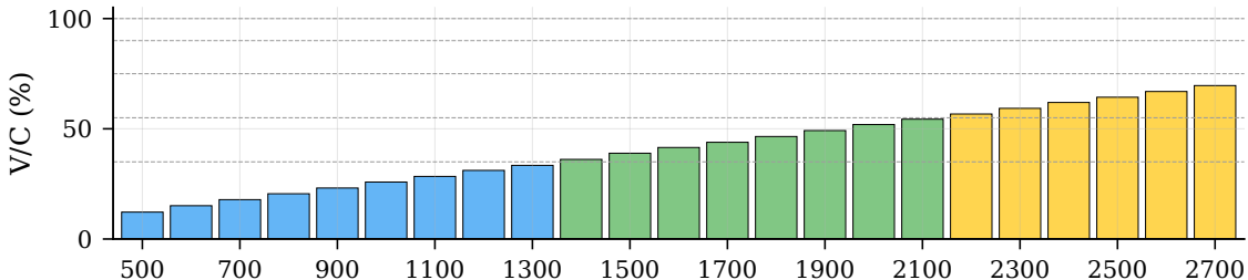
Demand 500-2700 veh/hr
