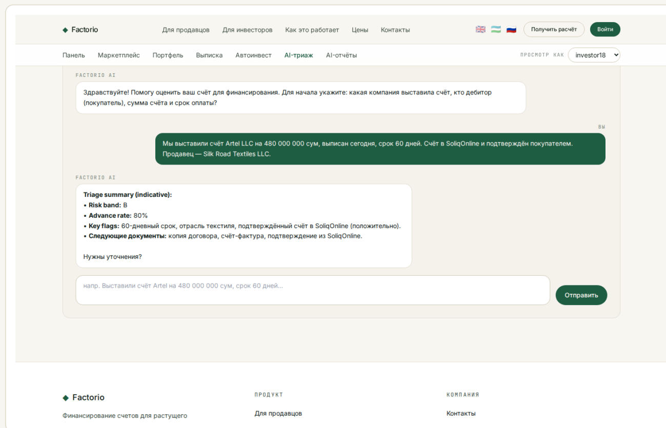
Действующий триаж счёта в чате в приложении Factorio
