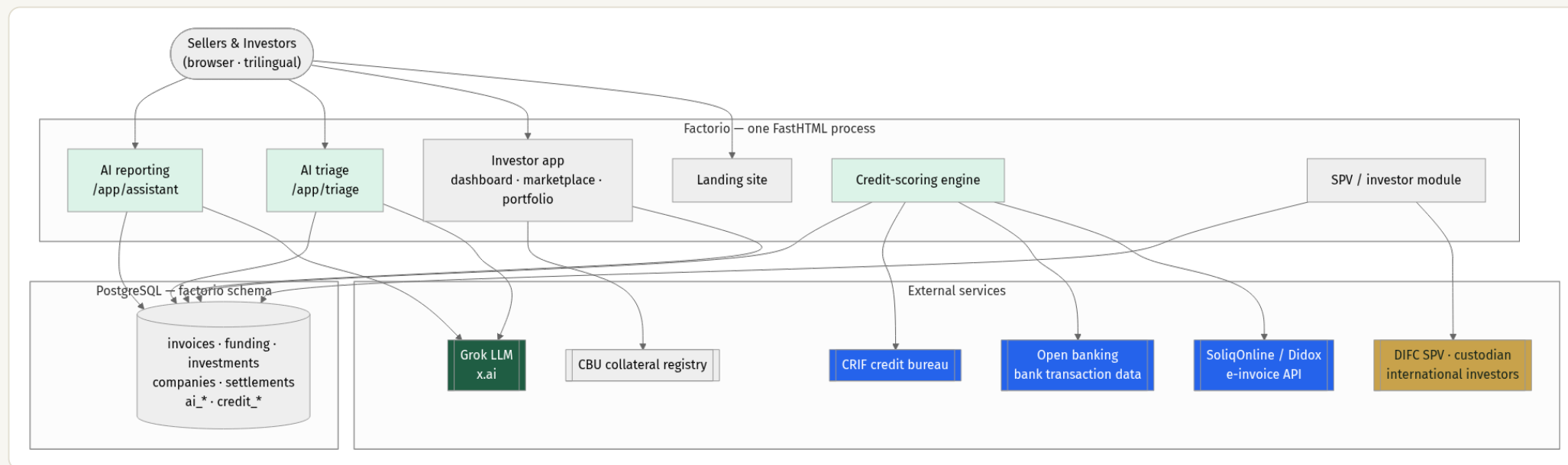
Целевая архитектура системы с выделенными ИИ-компонентами
