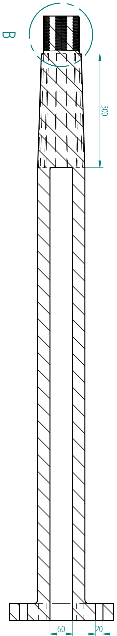
SECTION A-A
