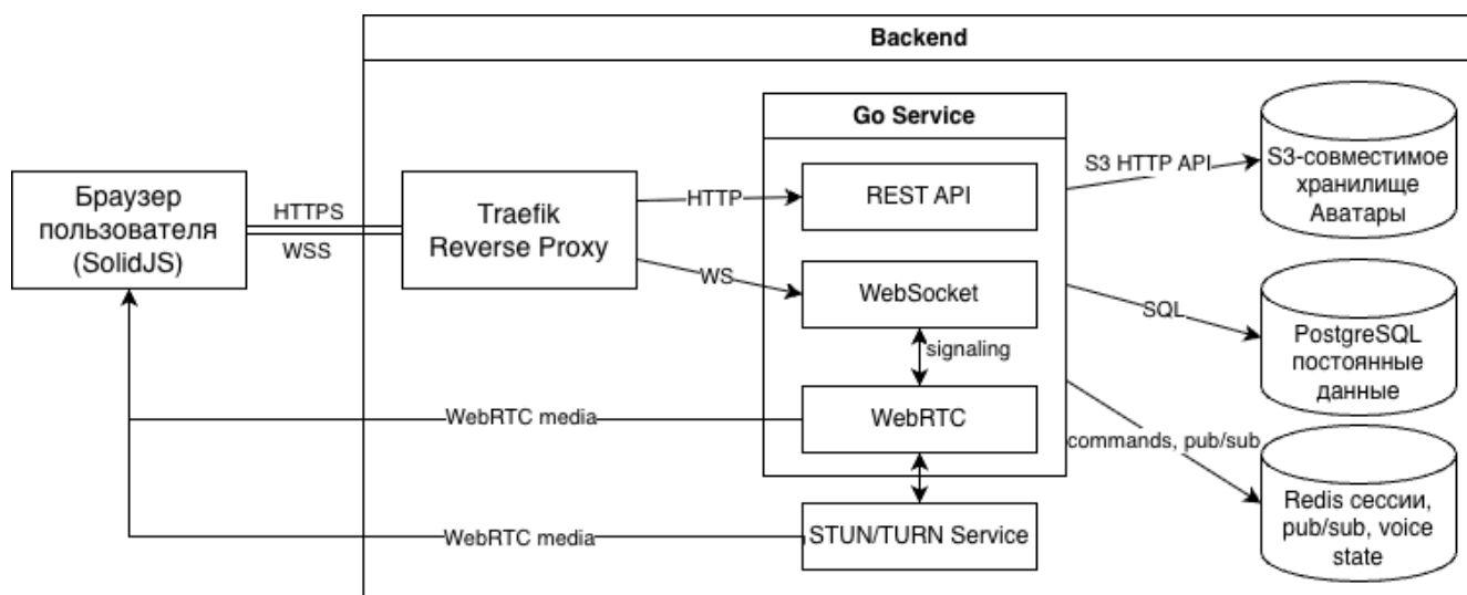
Рис. 4.1: Общая архитектура веб-приложения Chatterly
