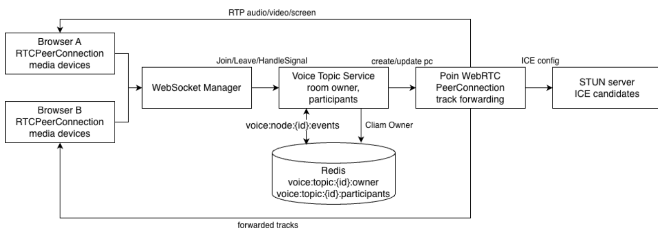
Рис. 4.5: Архитектура голосового топики и WebRTC-сигнализация
