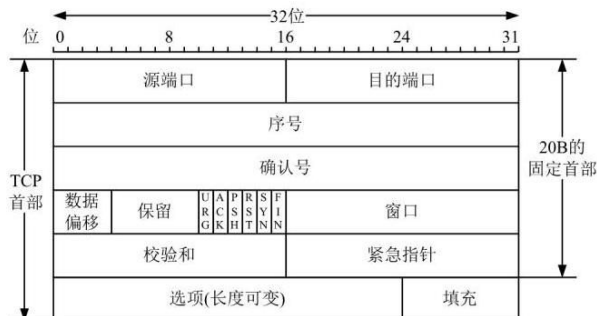
图2 TCP段头结构
