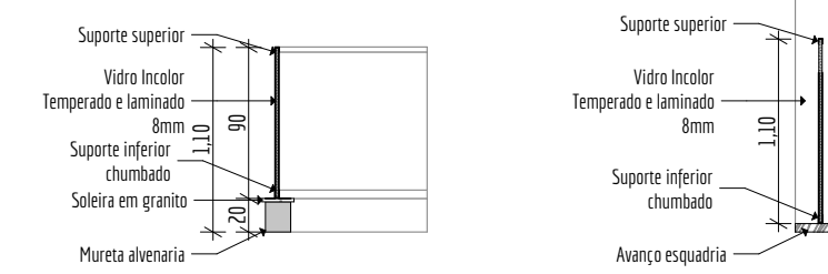
Guarda Corpo Escala: 1:50
