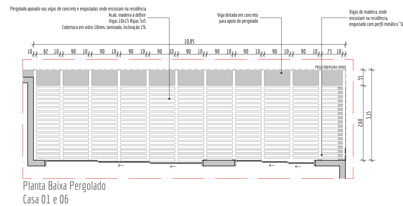
5 PERGOLADOS MADEIRA Escala: 1:75
