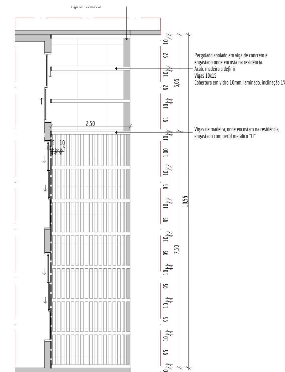
Planta Baixa Pergolado Casa 03 e 04
