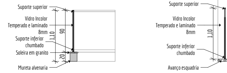
1 Guarda Corpo Escala: 1:50
