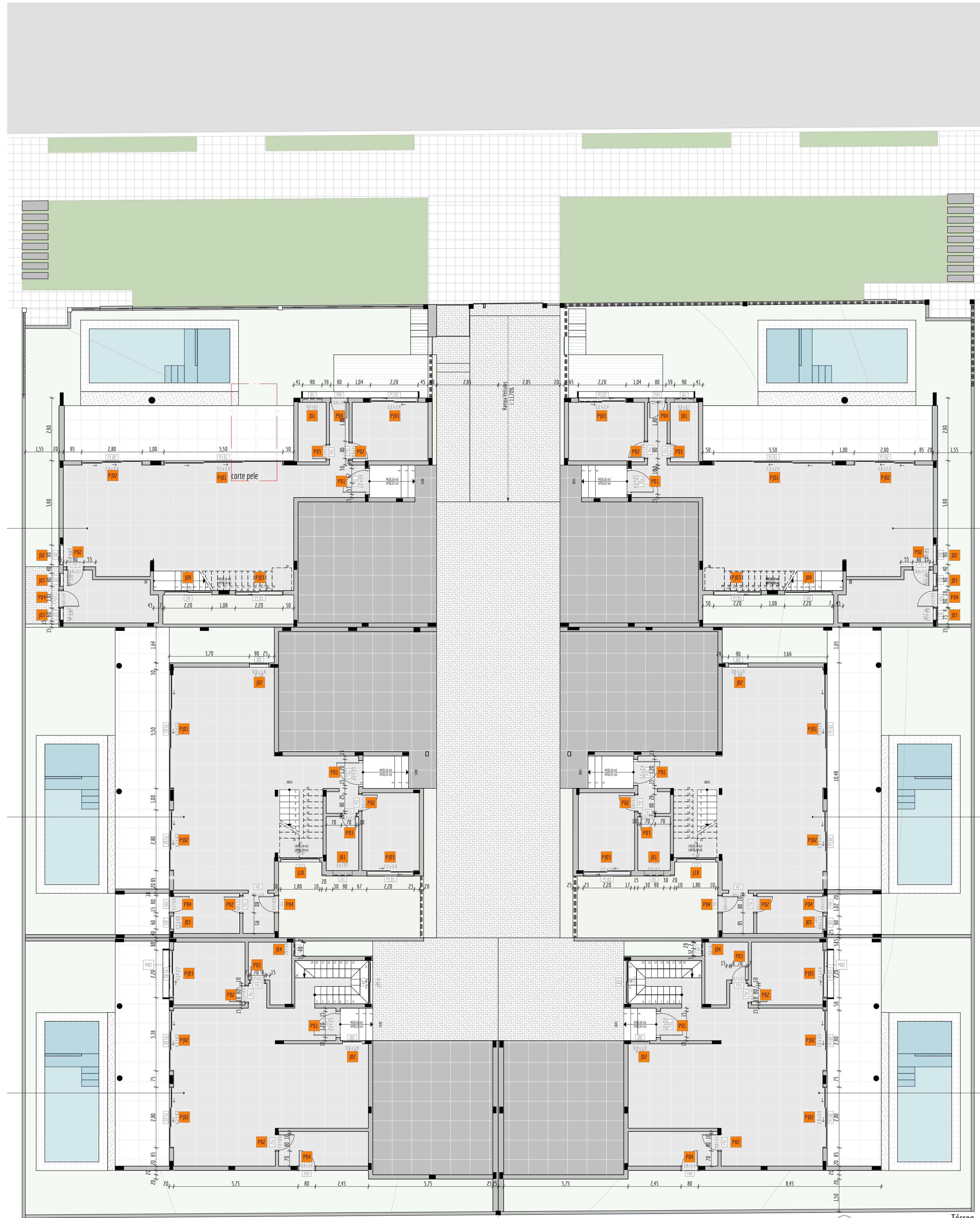
Térreo Escala: 1:100
