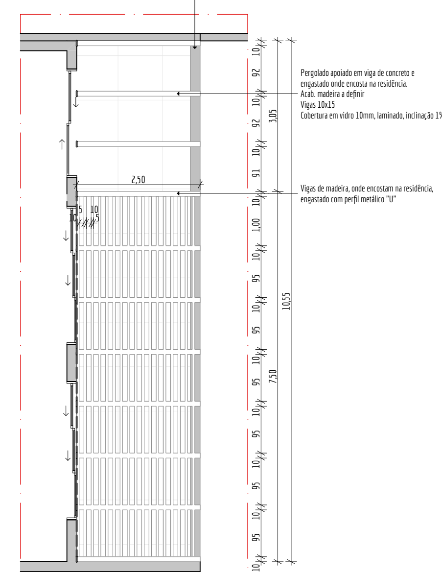
Planta Baixa Pergolado Casa 03 e 04
