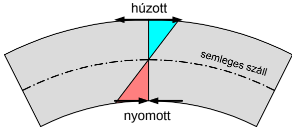
A hajlított tartó elmozdulásai
