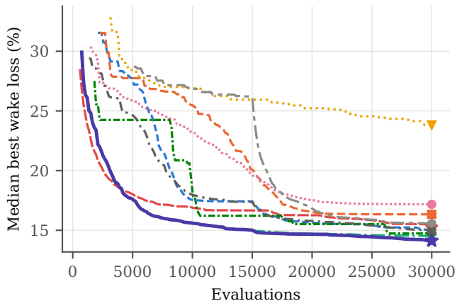
IEA37 CS1, 16 turbines, 30,030 evaluations
