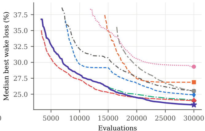
IEA37 CS1, 36 turbines, 30,030 evaluations
