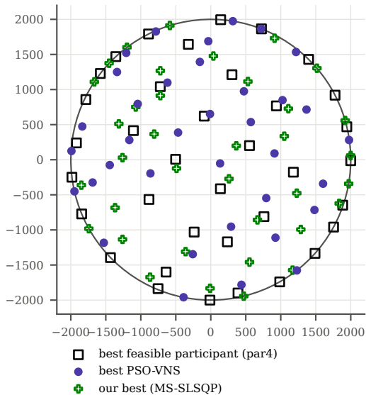
IEA37 CS1, 36 turbines (m)
