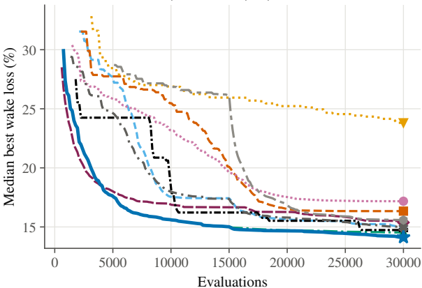
IEA37 CS1, 16 turbines, 30,030 evaluations
