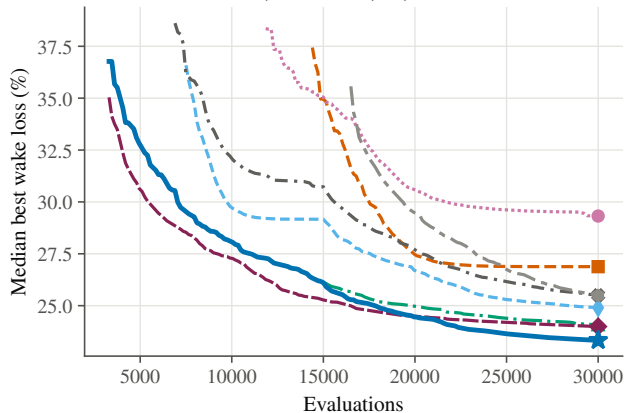
IEA37 CS1, 36 turbines, 30,030 evaluations
