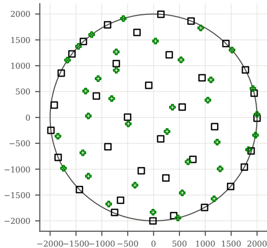
IEA37 CS1, 36 turbines (m)
