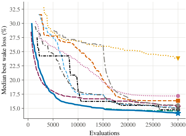
IEA37 CS1, 16 turbines, 30,030 evaluations
