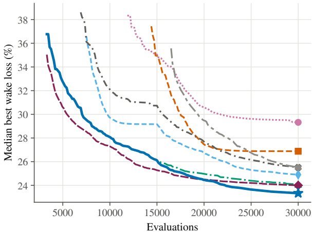
IEA37 CS1, 36 turbines, 30,030 evaluations
