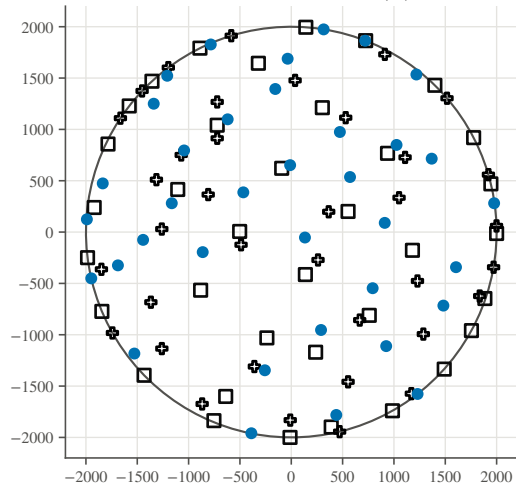
IEA37 CS1, 36 turbines (m)
