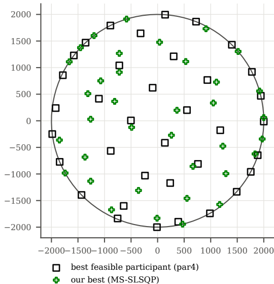
IEA37 CS1, 36 turbines (m)
