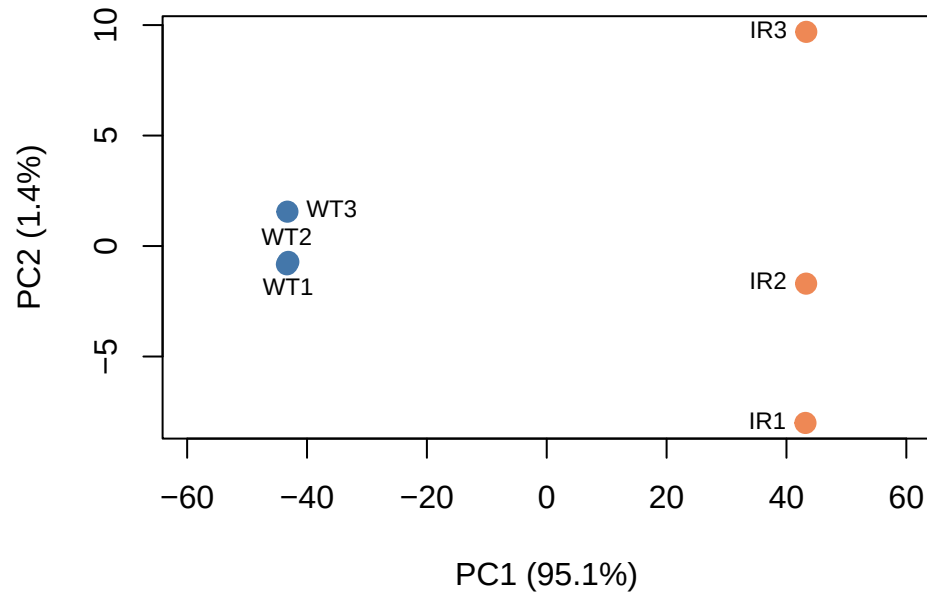
Unsupervised PCA
