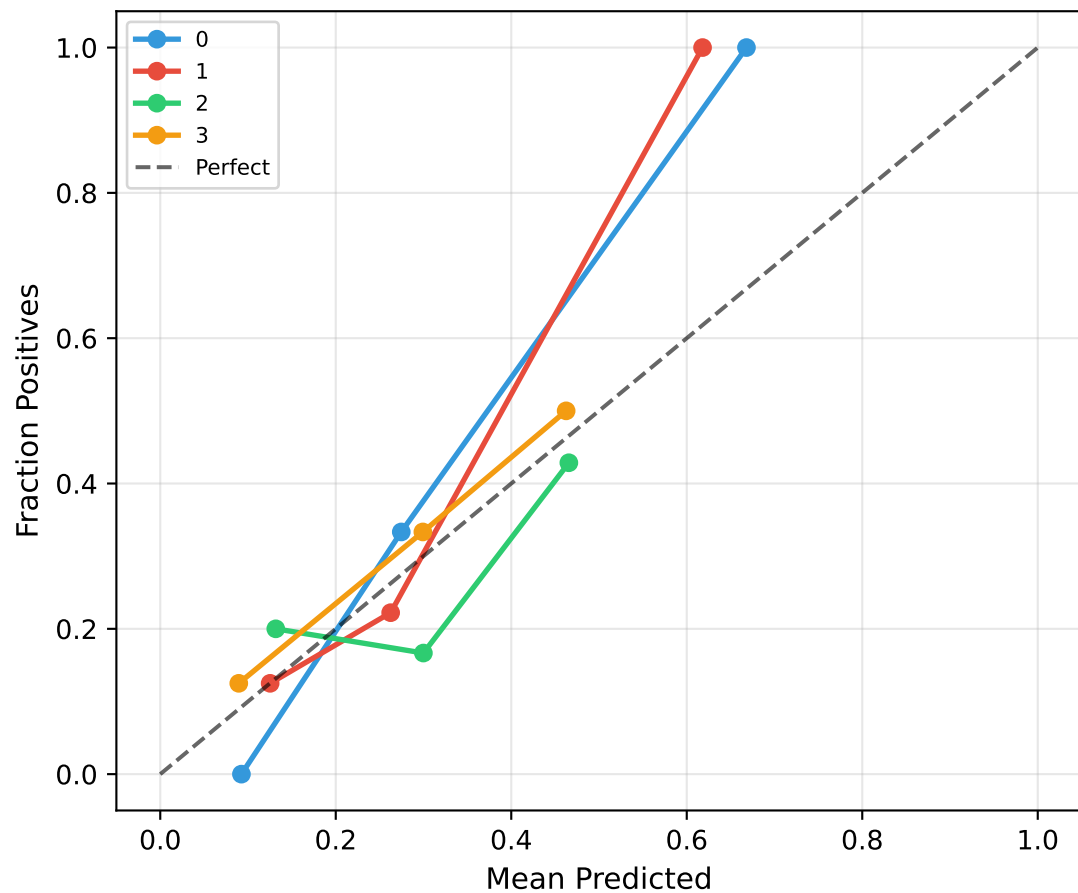
Calibration (RF)
