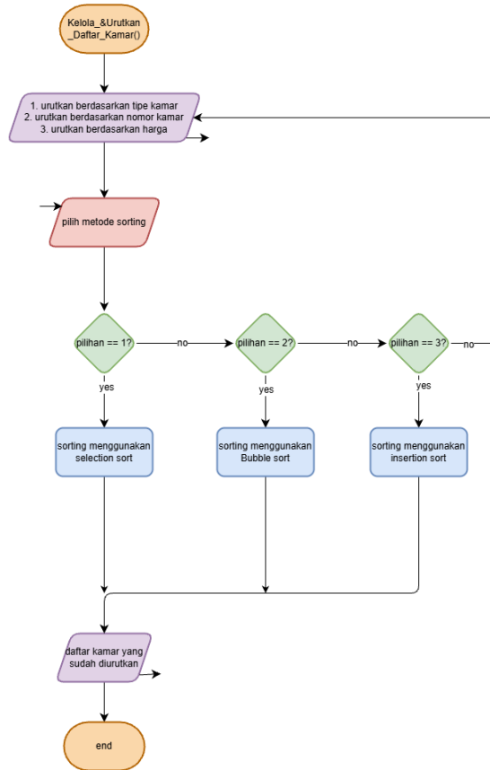
gambar 2.7 Flowchart Kelola dan urutkan daftar kamar
