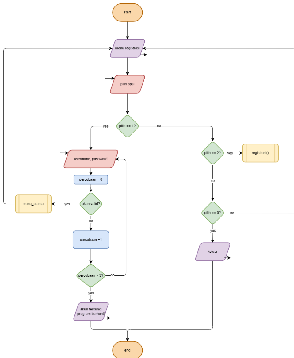
gambar 2.1 Flowchart menu Registrasi
