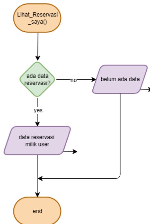
gambar 2.12 Flowchart lihat reservasi milik user
