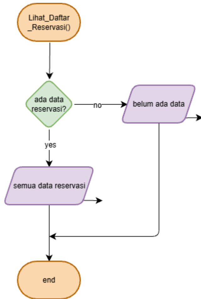
gambar 2.4 Flowchart Lihat Daftar Reservasi (Read)
