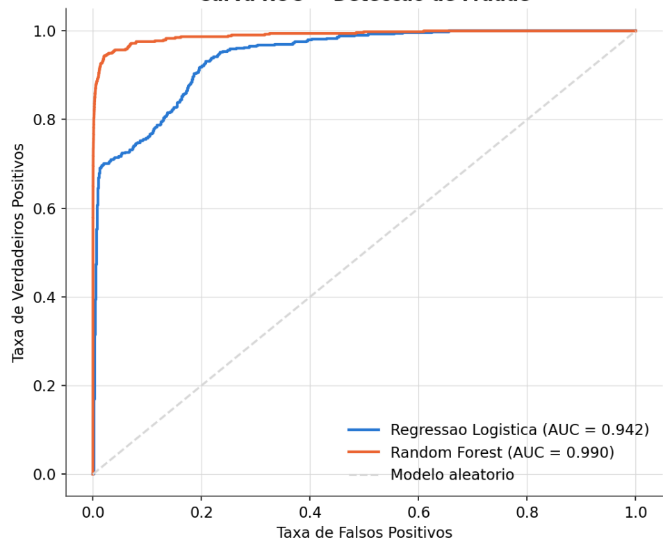
Curva ROC — Deteccao de Fraude
