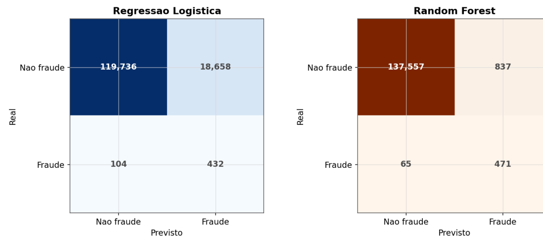
Matriz de Confusao — Conjunto de Teste
