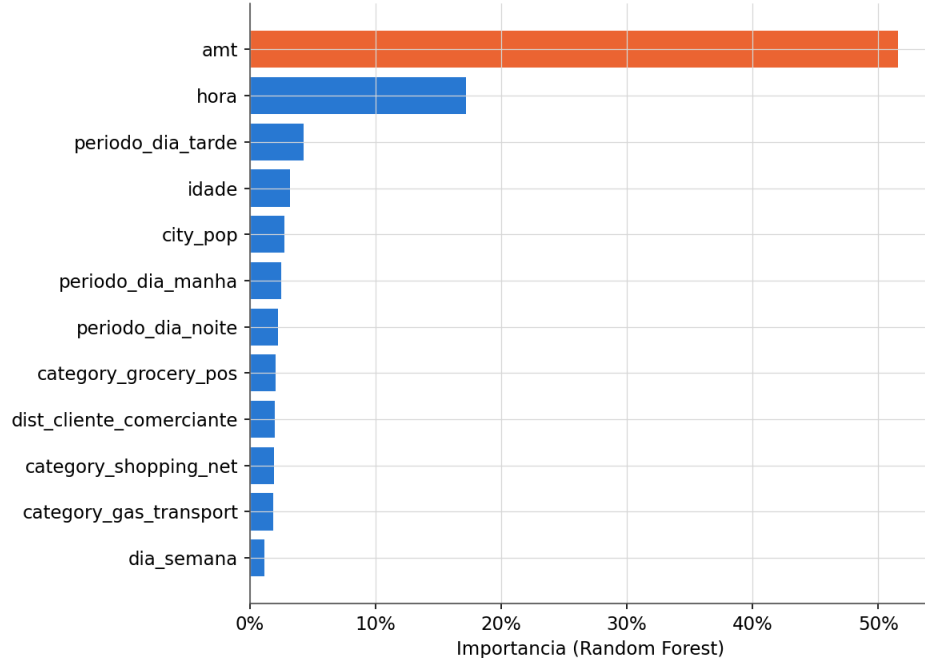
Variáveis Mais Relevantes para Detectar Fraude
