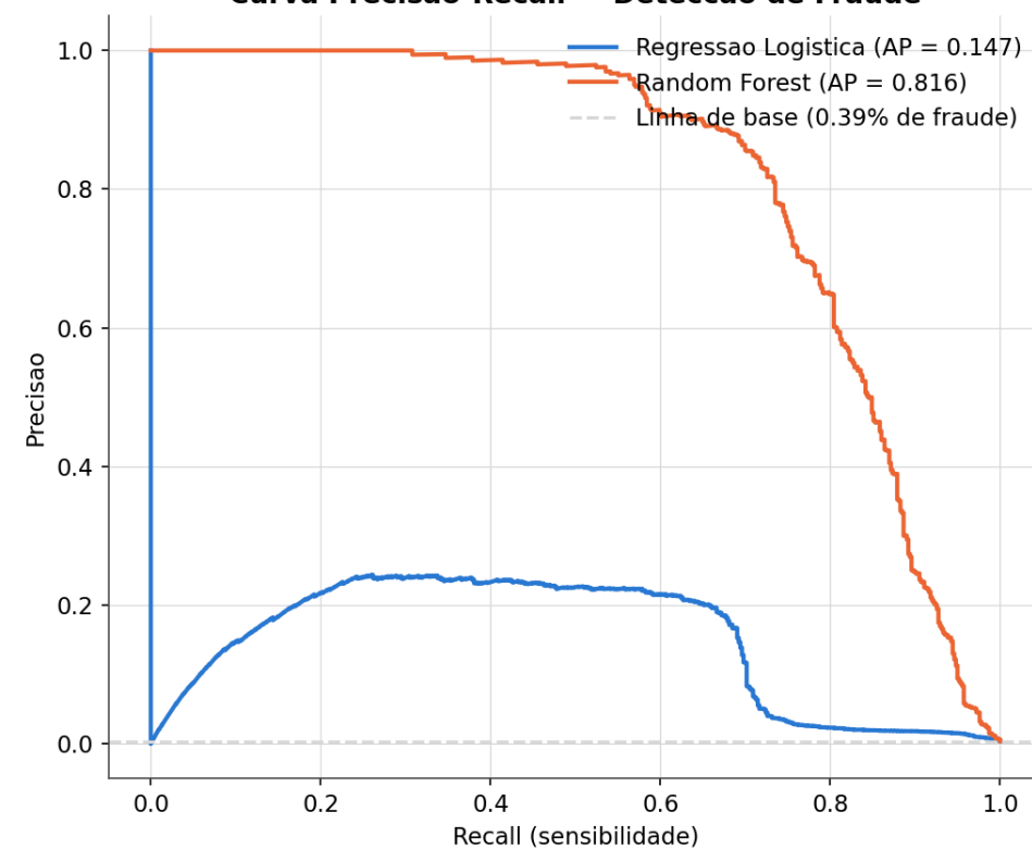
Curva Precisao-Recall — Deteccao de Fraude
