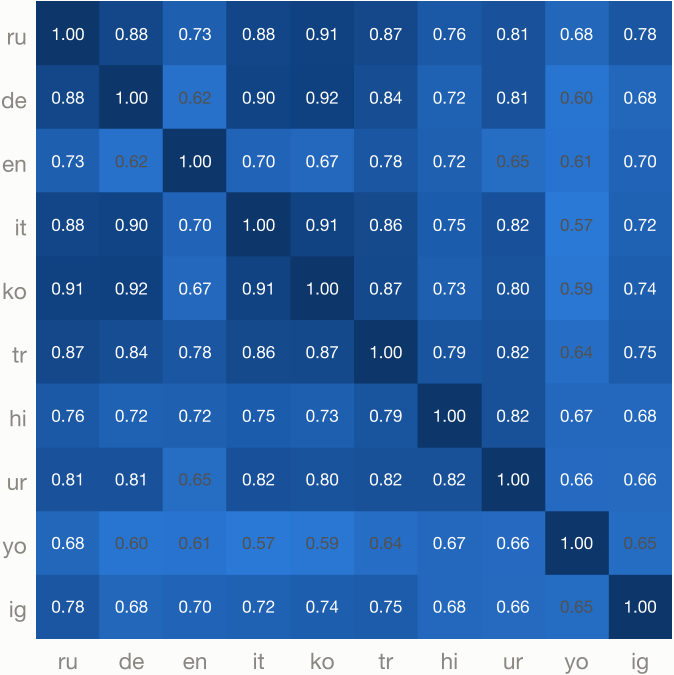
Llama-3.1-8B-Instruct · layer 8
