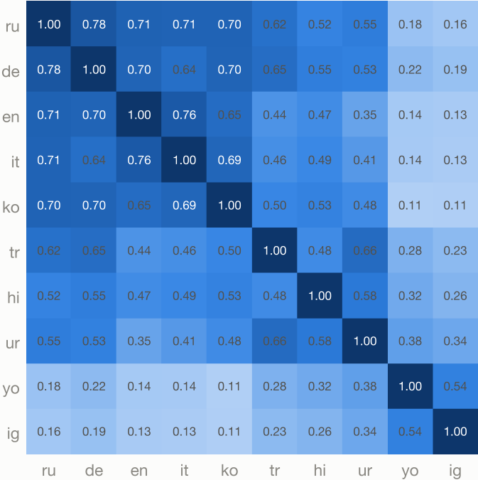
Qwen3-8B · layer 20
