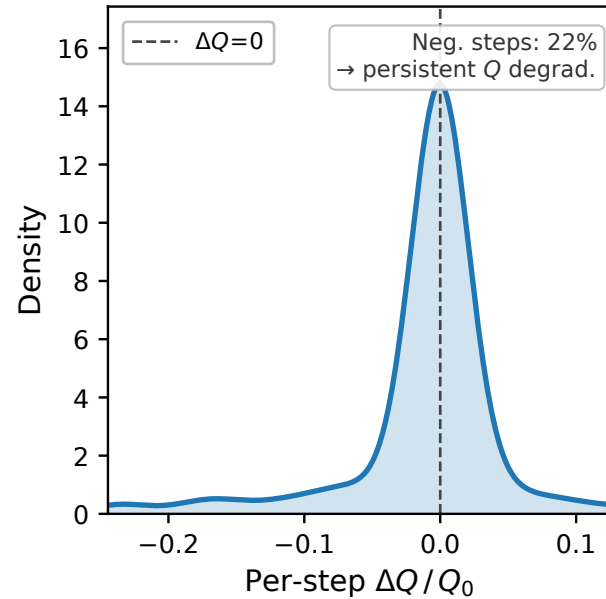
(d) Per-step \Delta Q KDE
