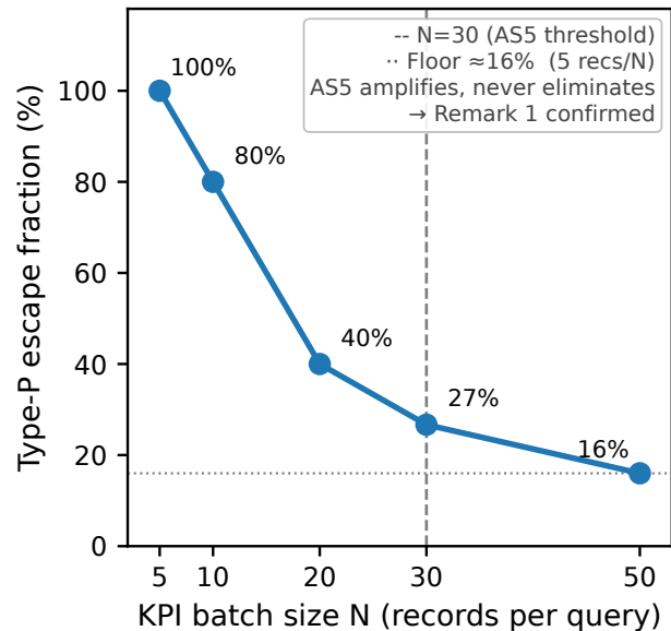
(d) AS5 amplifies via batch size N
